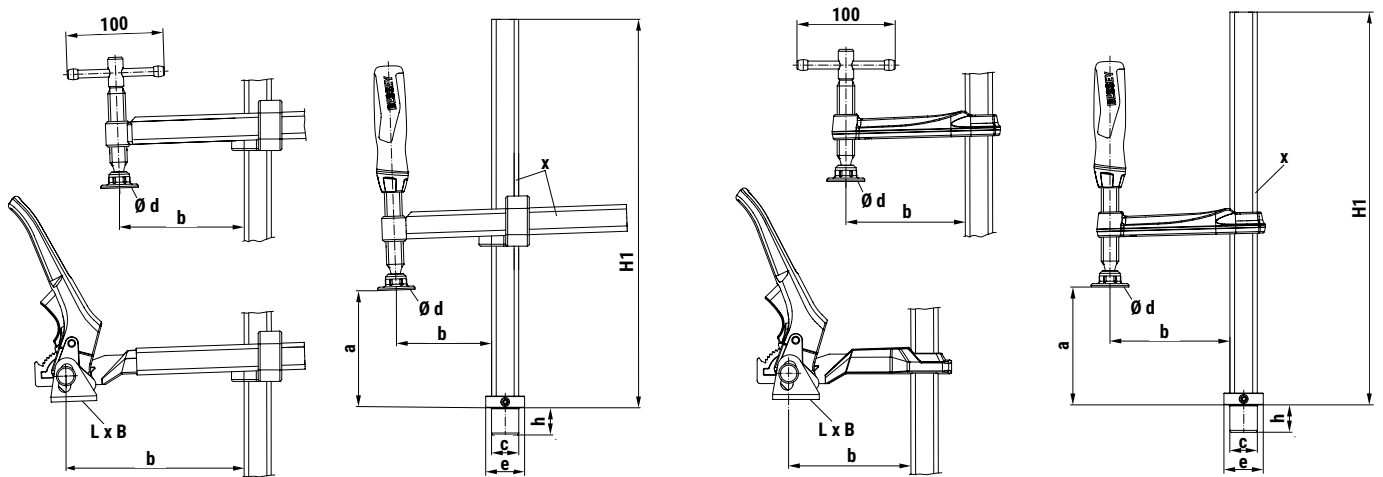
Maßtabelle TWV16 / TW16 / TW22
